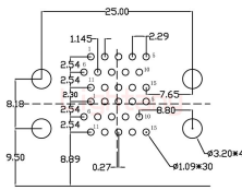
PCB布局 (PCB Layout)
